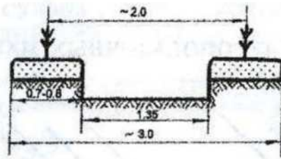
Плуг лесной полостный ПЛП-135
