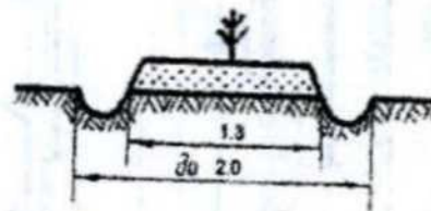
Плуг лесной ПЛМ-1.3
