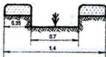
Плуг комбинированный лесной ПКЛ-70-4 (двухотвальный)
