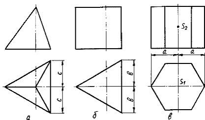
Рисунок 41. Изображение плоскостей симметрии
